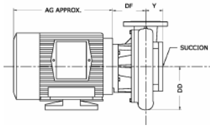
AZ MONOBLOCK
